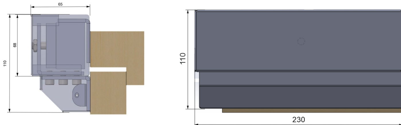
Рисунок 1. Габаритные размеры
